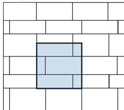
80 x 50 x 7,5 cm - environ 1 pces/m 2 80 x 40 x 7,5 cm - environ 1,5 pces/m 2 80 x 30 x 7,5 cm - environ 1,5 pces/m 2
