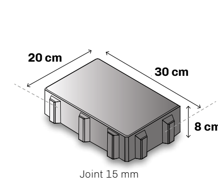
POSE À JOINTS DROITS
