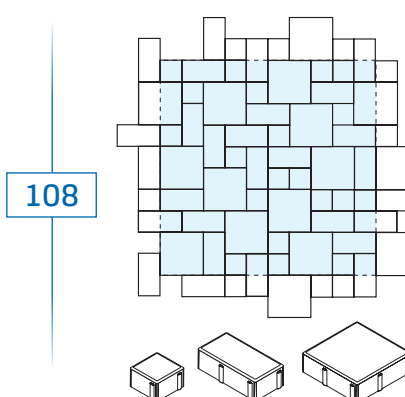
10 x 10 x 6 / 8 - environ 20 pièces/m 2 10 x 20 x 6 / 8 - environ 18 pièces/m 2 20 x 20 x 6 / 8 - environ 11 pièces/m 2
