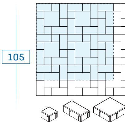
10 x 10 x 6 / 8 - environ 25 pièces/m 2 10 x 20 x 6 / 8 - environ 25 pièces/m 2 20 x 20 x 6 / 8 - environ 6,25 pièces/m 2
