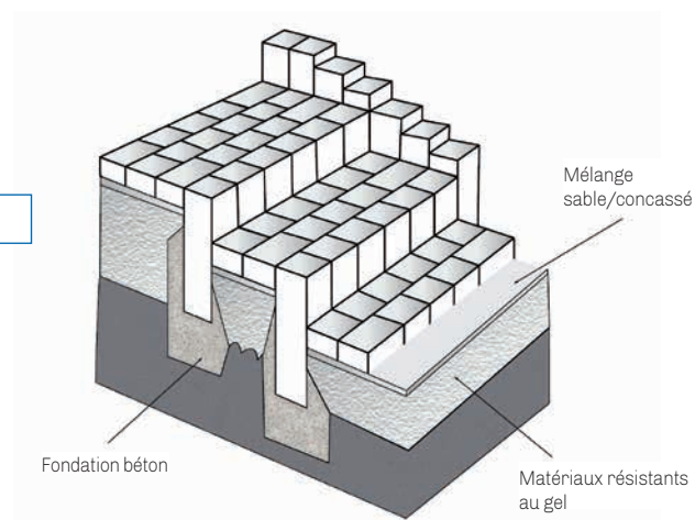
Réalisation d'un escalier en palissades et pavés
