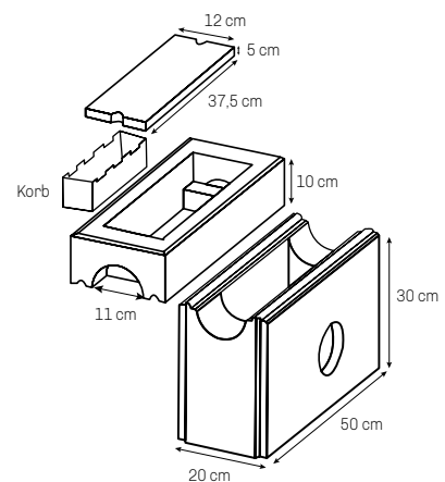
Entwässerungsschacht
