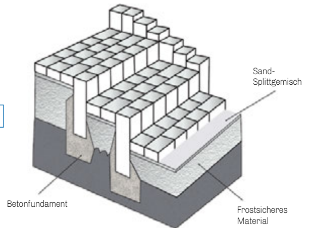
Einbau von Palisaden und Pflaster als Stellstufen
